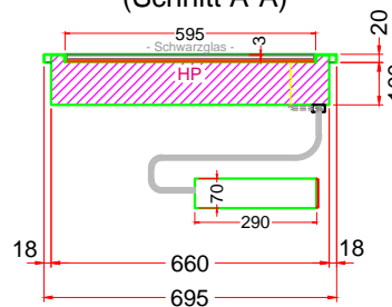
(Schnitt A-A)
